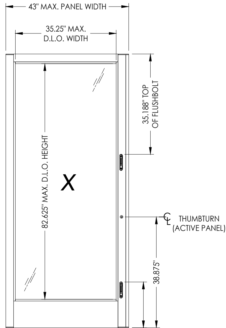
DOOR PANEL
